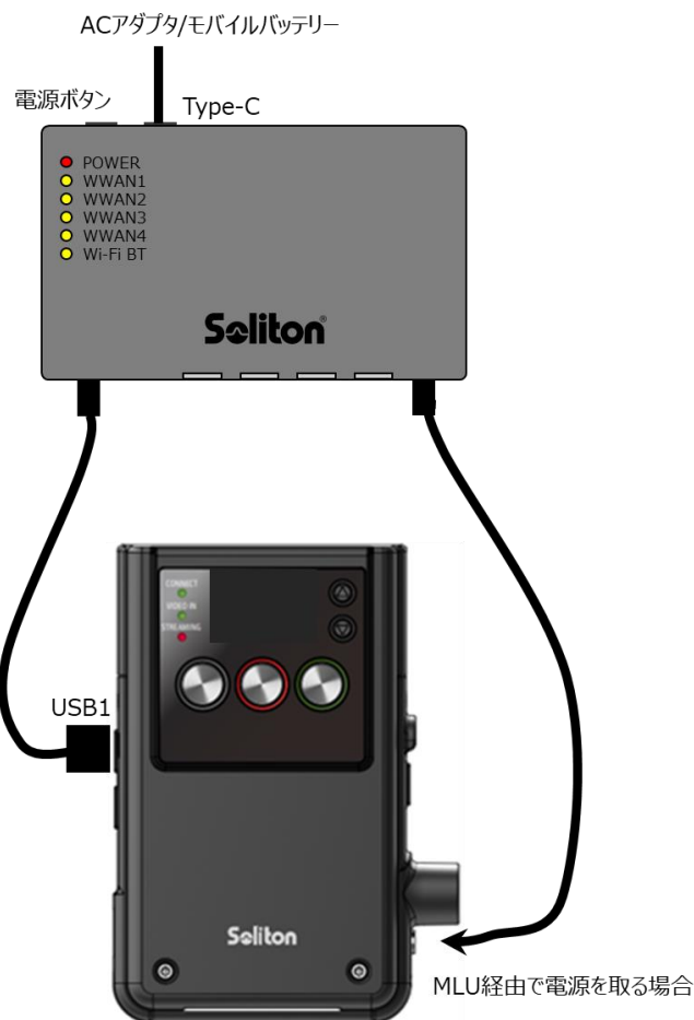
図 1-4 MLU と Zao-X の接続
